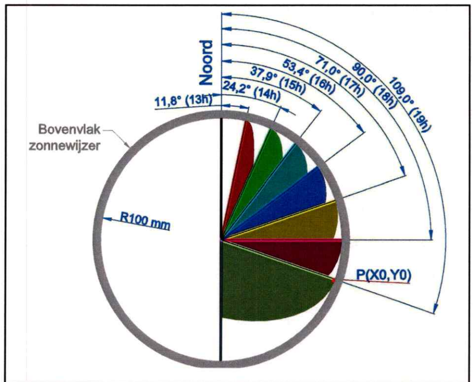
Fig. 3: Hoekmaat voor de markeerschijven van 13h-19h zonnetijd.
