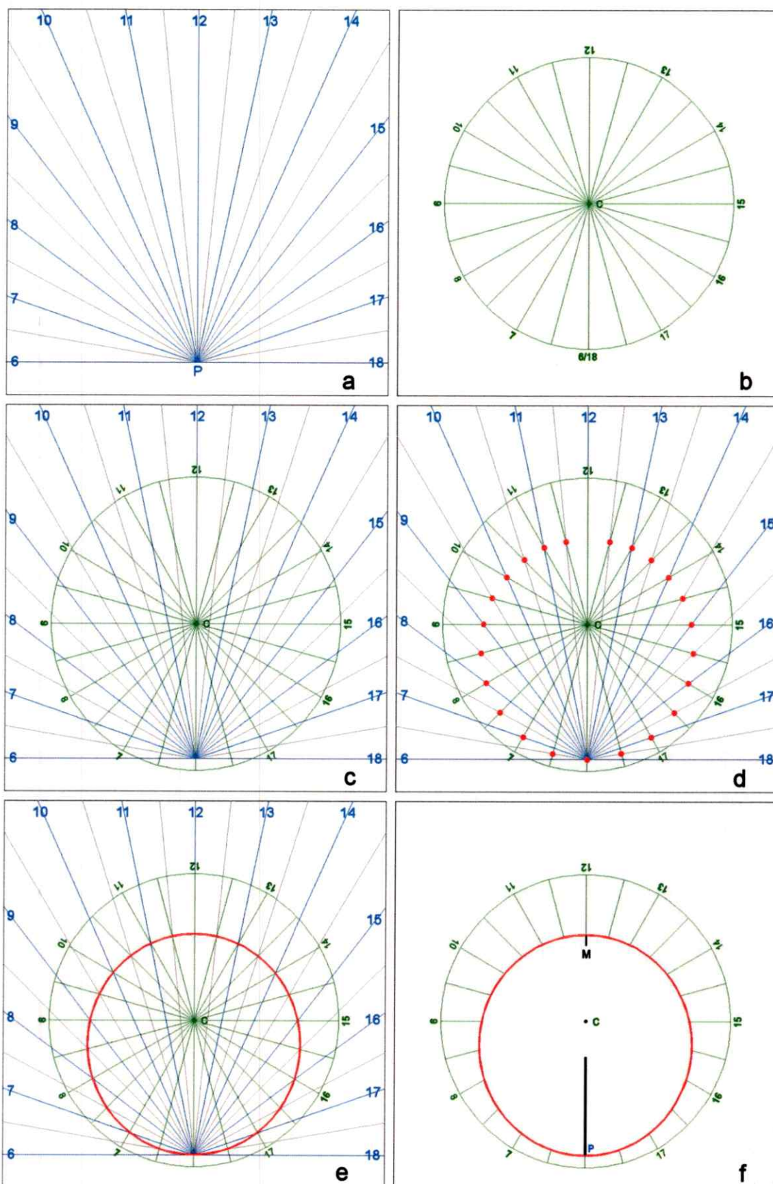
Fig. 5. De constructie van de Sawyer Equant zonnemijzer. a. Horizontale zonnemijzer voor 51^{\circ} 10' . Uurlijnen in blauw van 6 tot 18 uur, halfuurlijnen in grijs. P is het voetpunt van de poolstijl. b. Cirkel met middelpunt C, verdeeld in 12 uren van 30^{\circ} , met halfuurlijnen, in groen. c. De cirkel wordt op de zonnemijzer gelegd, met punt C op de 12-uurslijn. d. De snijpunten van de overeenkomstige uur- en halfuurlijnen worden gemarkeerd in rood. e. De rode punten worden verbonden door een vloeiende kromme. f. De uurlijnen van fig. 5a zijn verwijderd. De schaduwgever staat op de dikke lijn vanuit voetpunt P. De tijdscorrectie wordt ingesteld bij het merkpunt M.
