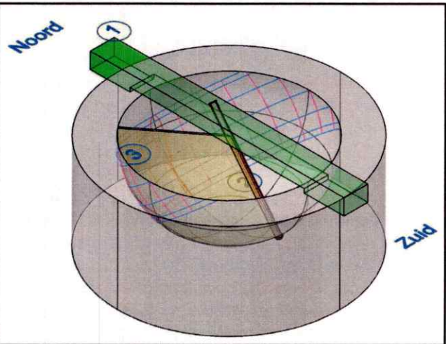
Fig. 5: Markeerinrichting.
