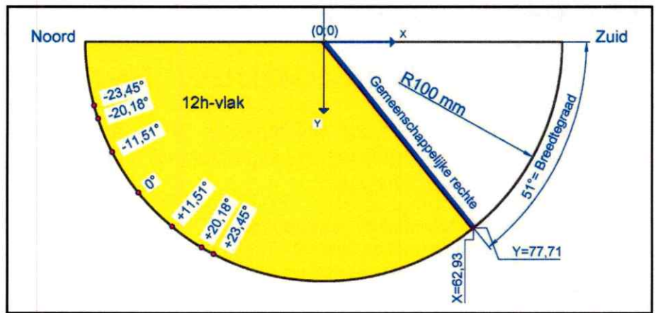
Fig. 2: Gemeenschappelijke snijlijn zonnetijdvlakken.
