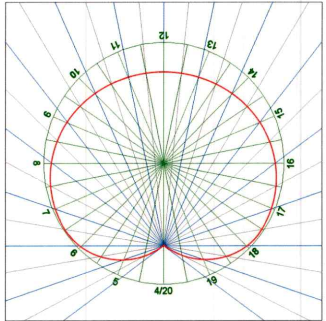
Fig. 7. De constructie van de Sawyer Equant zonnewijzer voor een groter bereik. Vergelijk deze figuur met fig. 5e. De horizontale zonnewijzer heeft uurlijnen van 4 tot 20 uur (blauw); daarop een urencirkel verdeeld in 16 uren van 22,5° (groen). De kromme die de snijpunten van de overeenkomstige uurlijnen verbindt (rood) is hartvormig.
